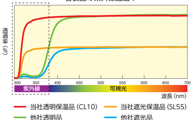
各製品の紫外線透過率
